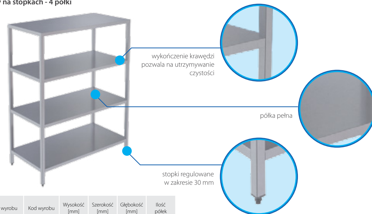
Regały na stopkach - 4 półki
